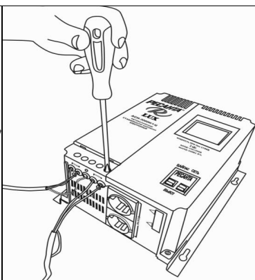
Рис 8. Подключение нагрузки
