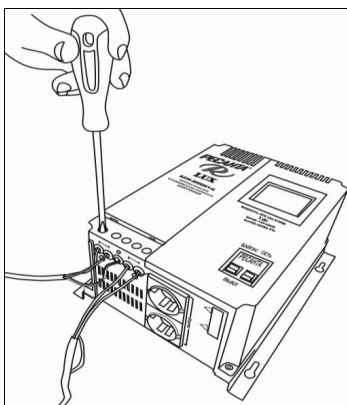
Рис 7. Подключение стабилизатора
