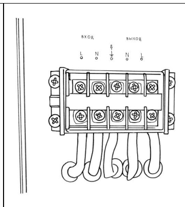
Рис. 6. Схема подключения
